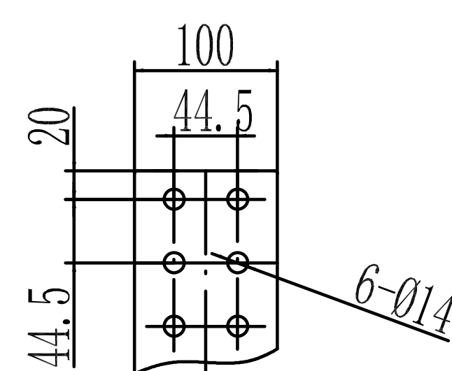
L. V. TERMINAL
