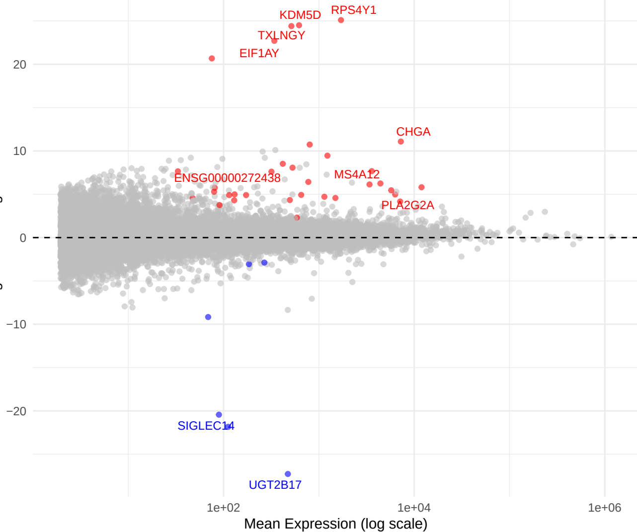
MA Plot: Villous Adenoma vs Tubular Adenoma
