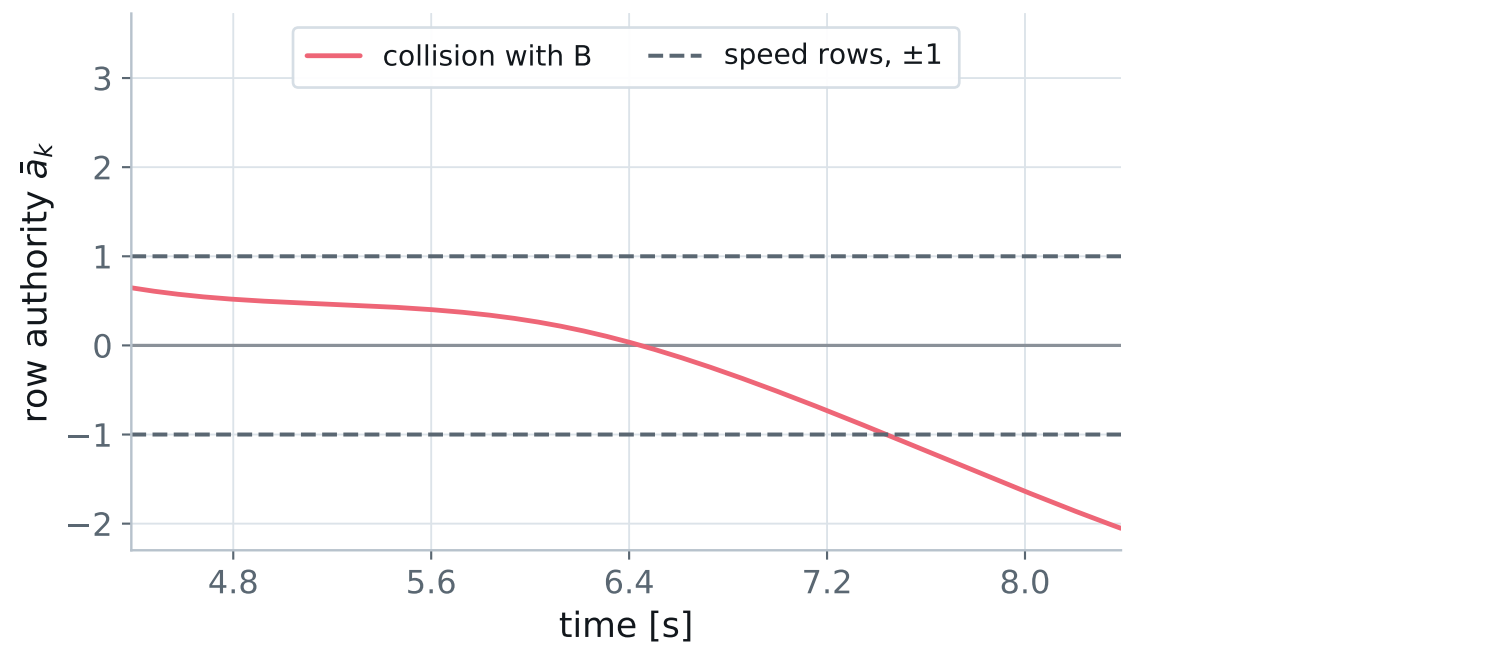
(d) agent A: collision authority crosses zero once per encounter
