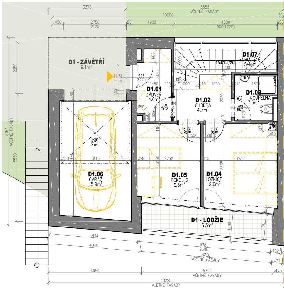
PŮDORYS 1.PP
