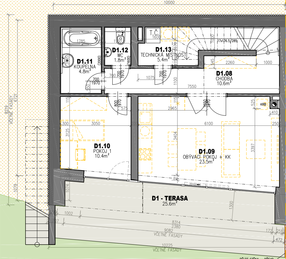
PŮDORYS 1.PP
