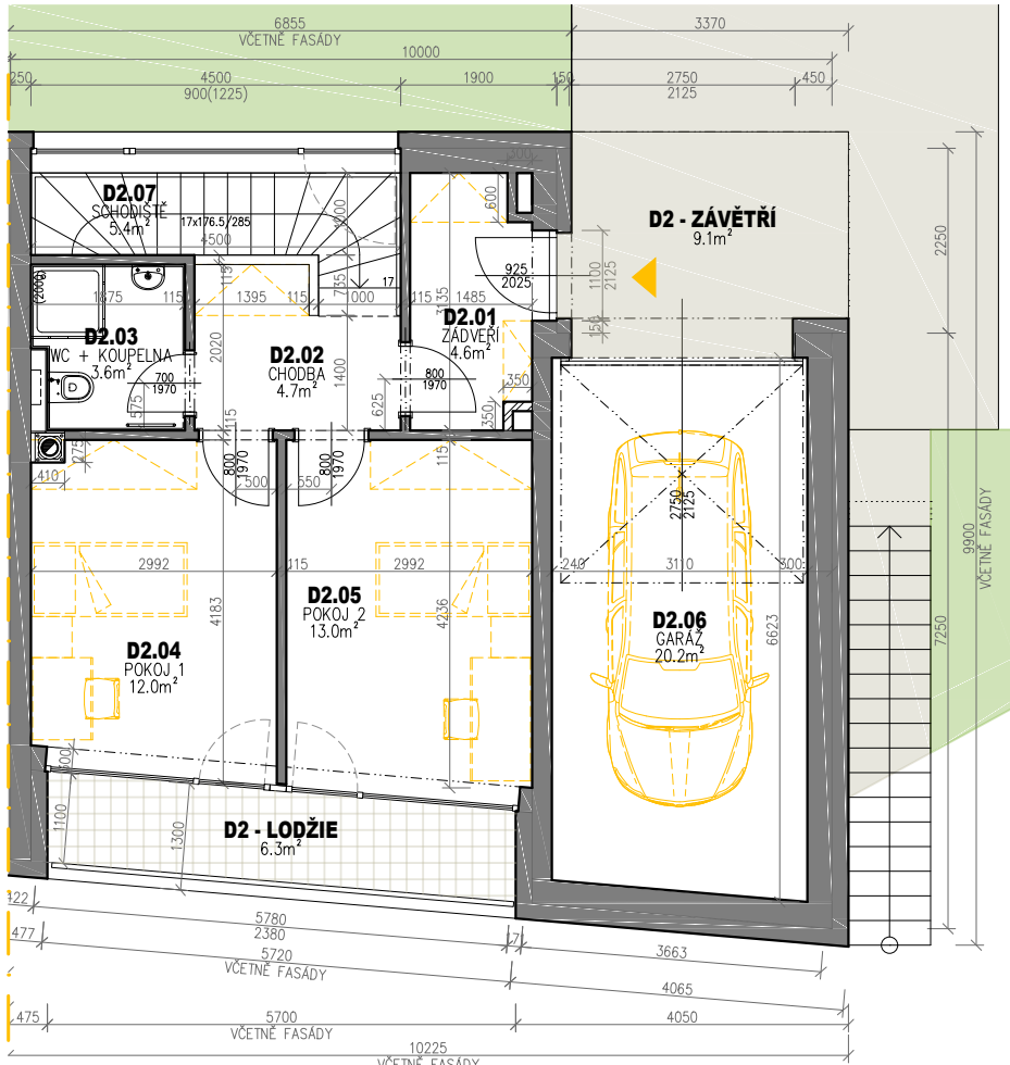
PŮDORYS 1.NP
