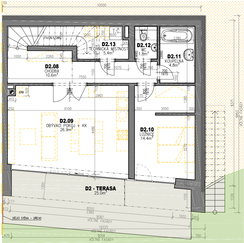
PŮDORYS 1.PP
