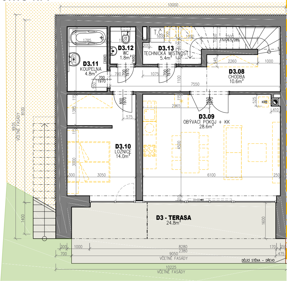
PŮDORYS 1.PP
