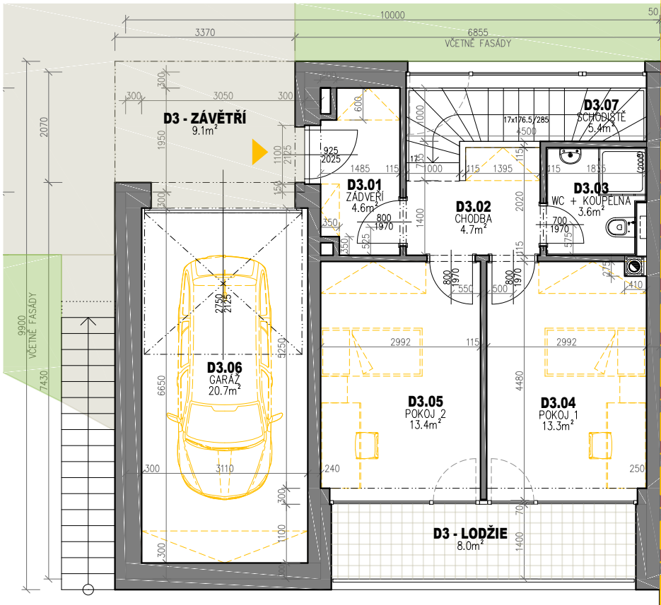
PŮDORYS 1.PP
