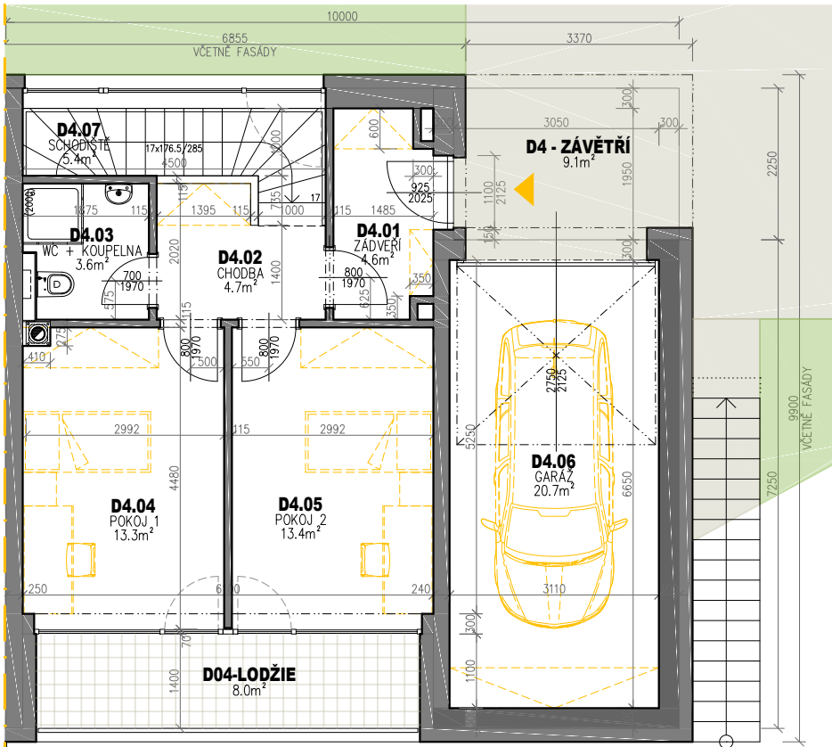
PŮDORYS 1.PP
