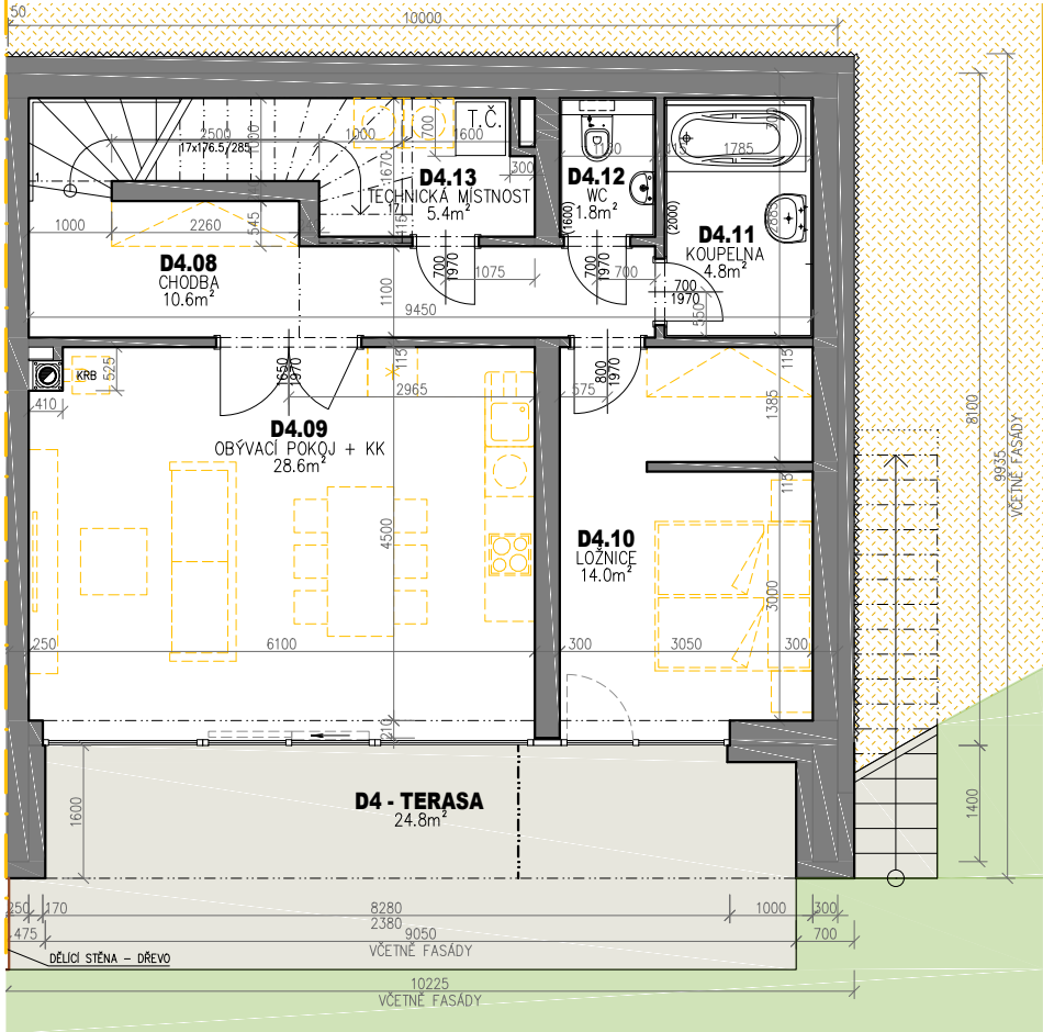
PŮDORYS 1.PP
