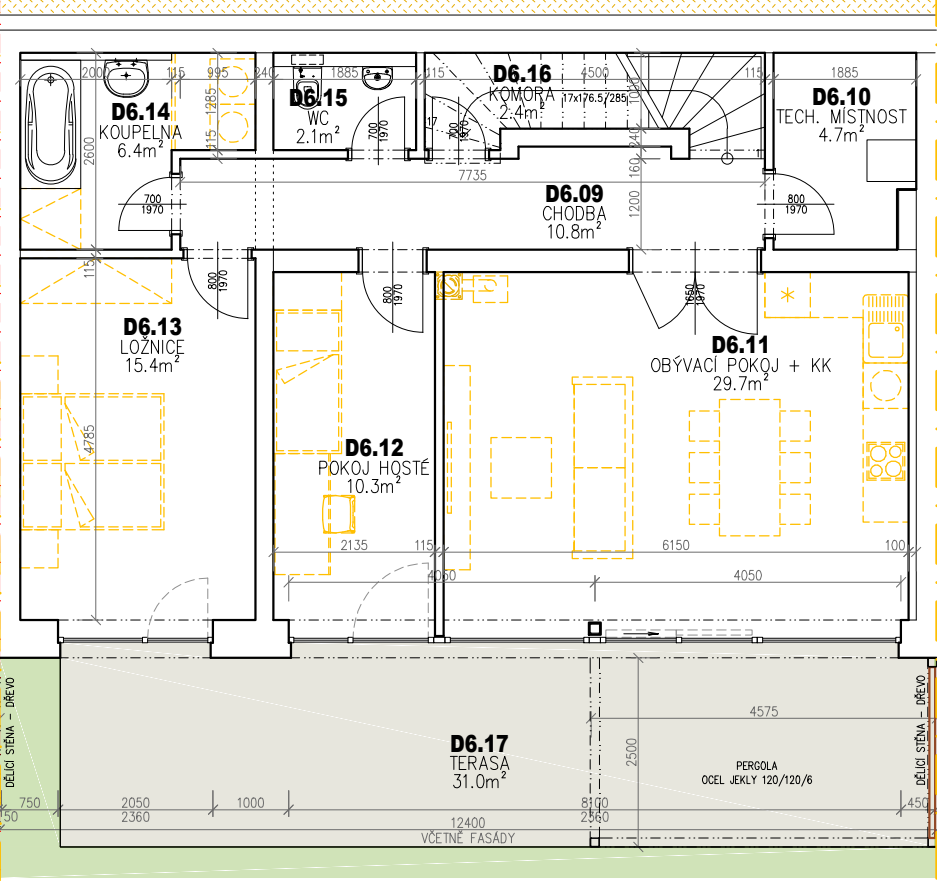
PŮDORYS 1.PP
