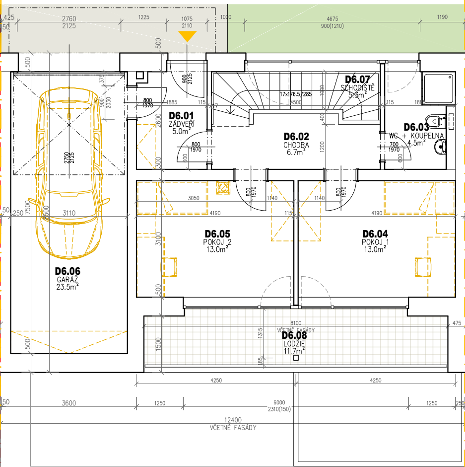
PŮDORYS 1.PP
