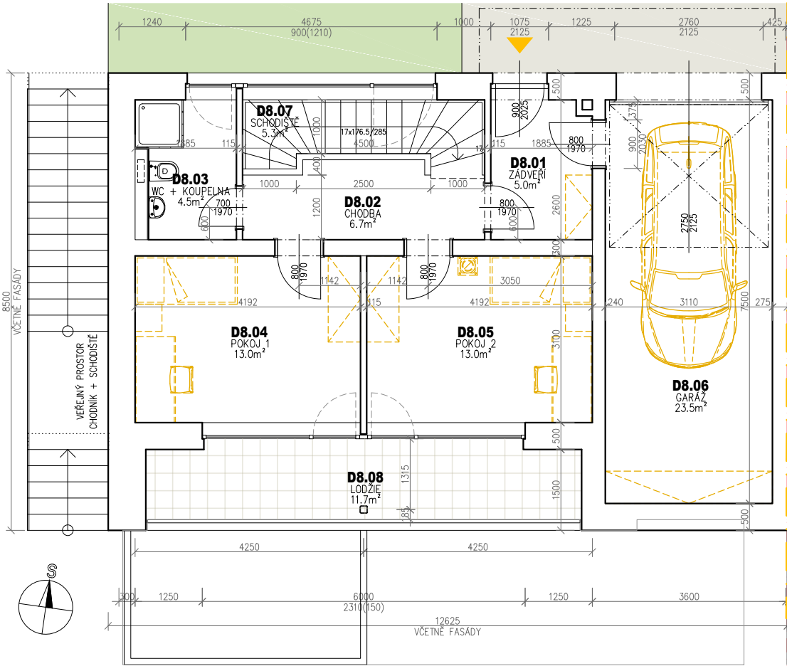
PŮDORYS 1.PP
