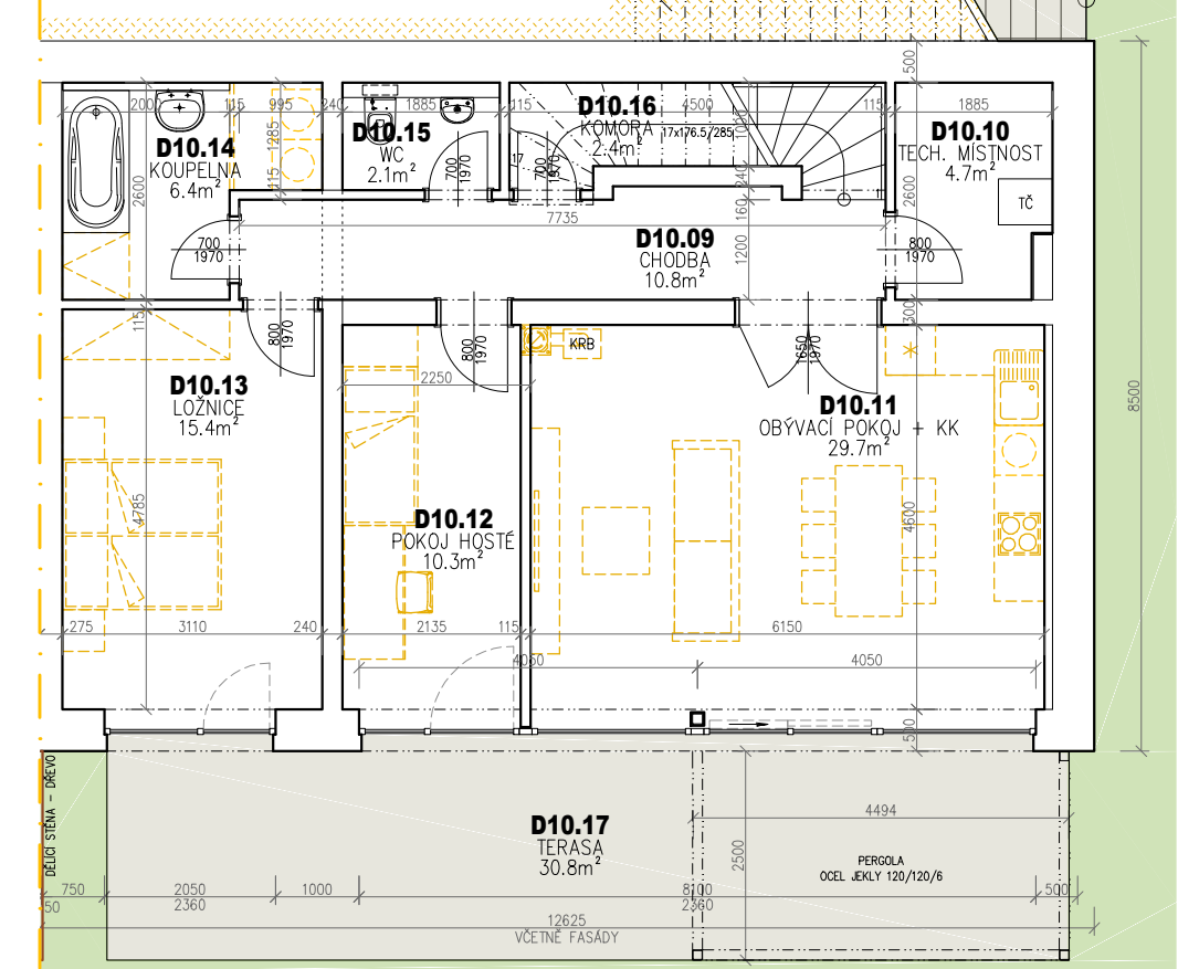
PŮDORYS 1.PP
