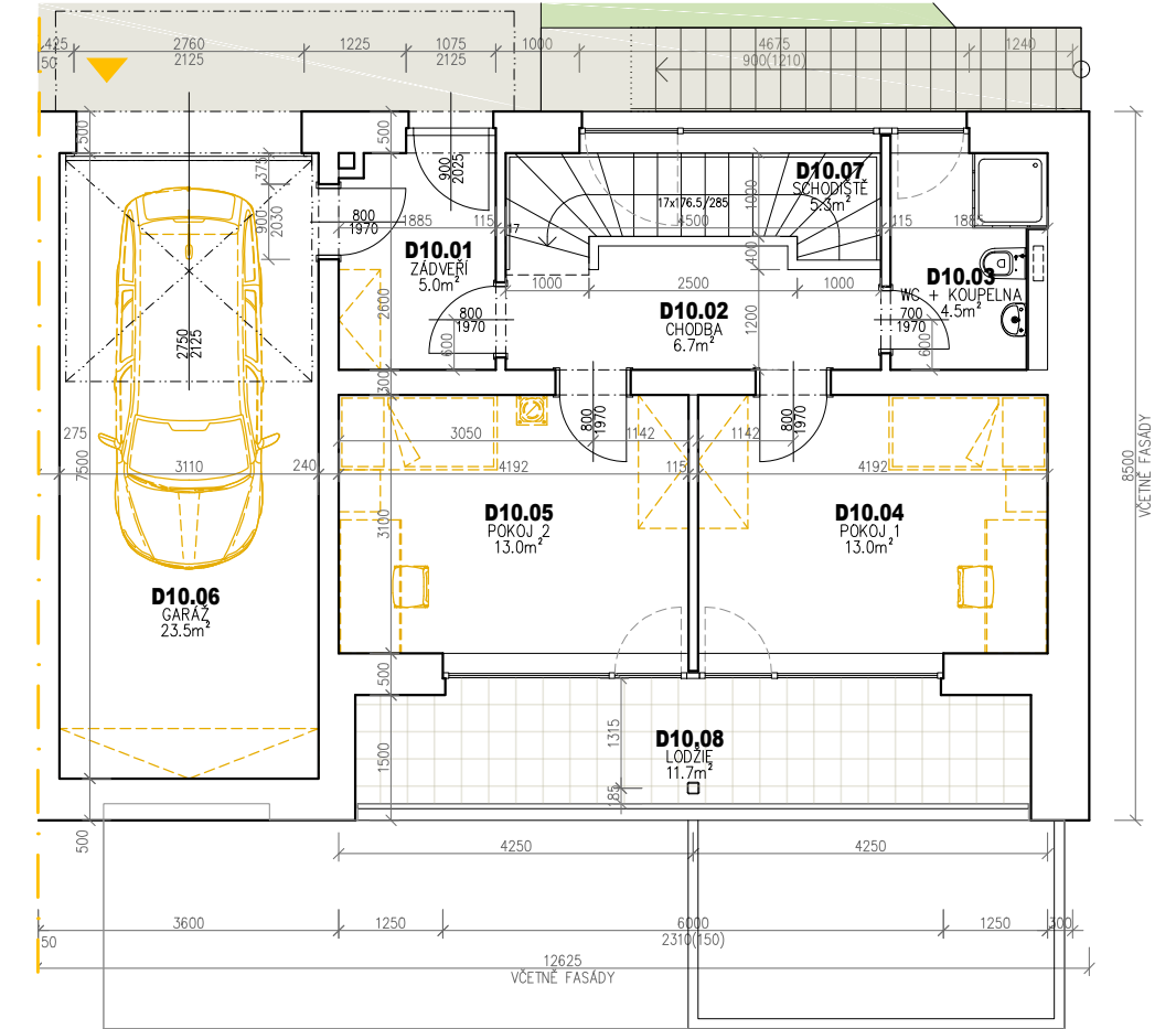
PŮDORYS 1.PP
