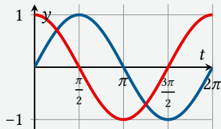
Sinus und Cosinus
