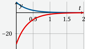
Exponentialfunktion
