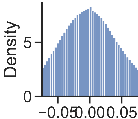
MobileNet-V2
