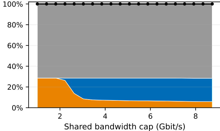
Bandwidth sweep Prefill fixed at 2.34 ktoken/s
