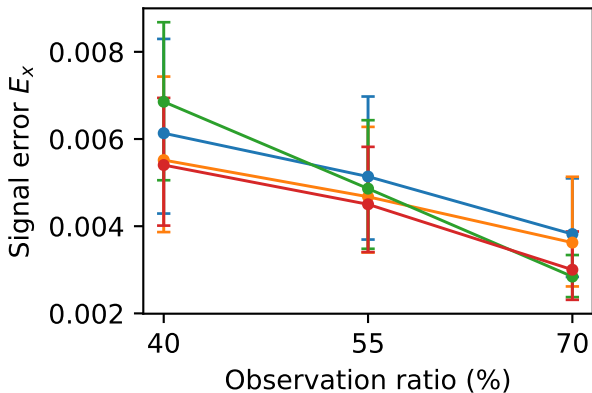
(d) Signal error E_x
