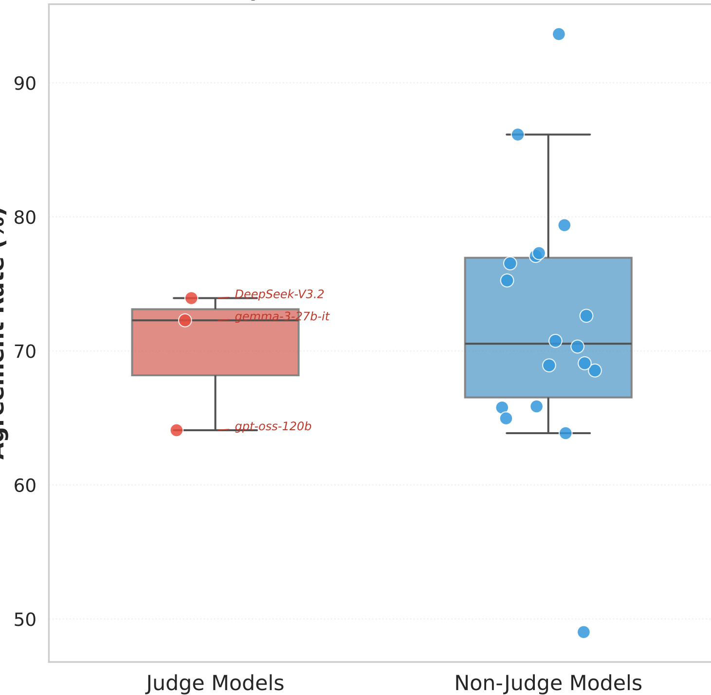
B Welch's t-test: p = 0.648 (n.s.)
