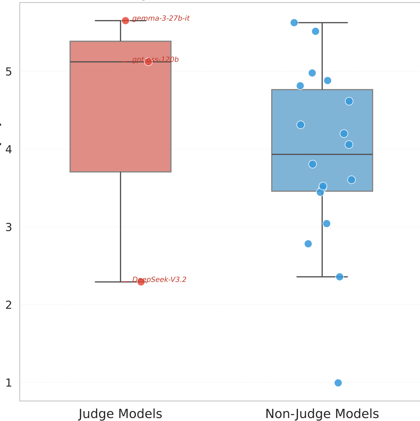
A Welch's t-test: p = 0.705 (n.s.)
