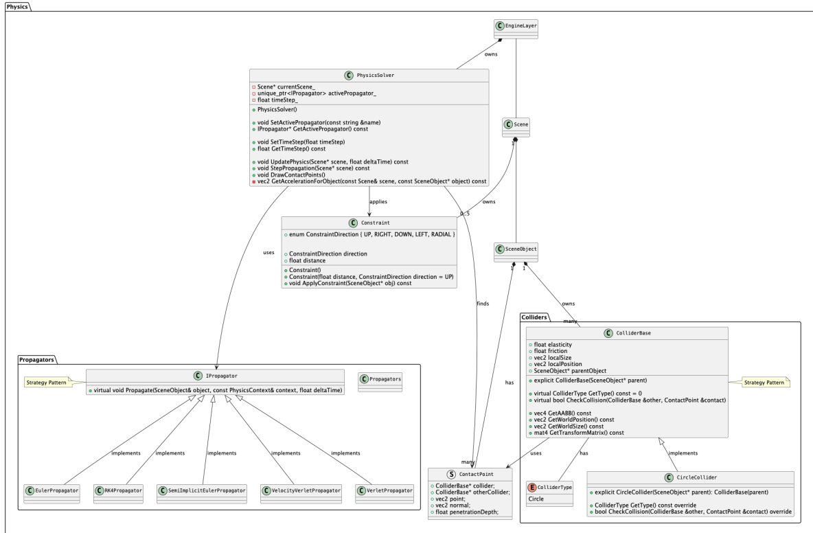
Abbildung 2: Überblick über die Struktur der Physik-Simulation, welche von der EngineLayer verwaltet wird
