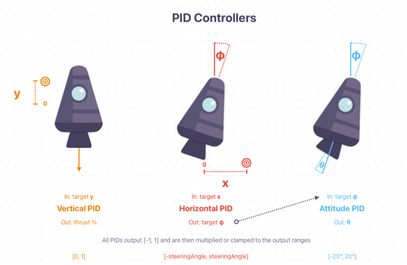
Abbildung 4: Regelungskonzept für die Schubvektor-kontrolle
