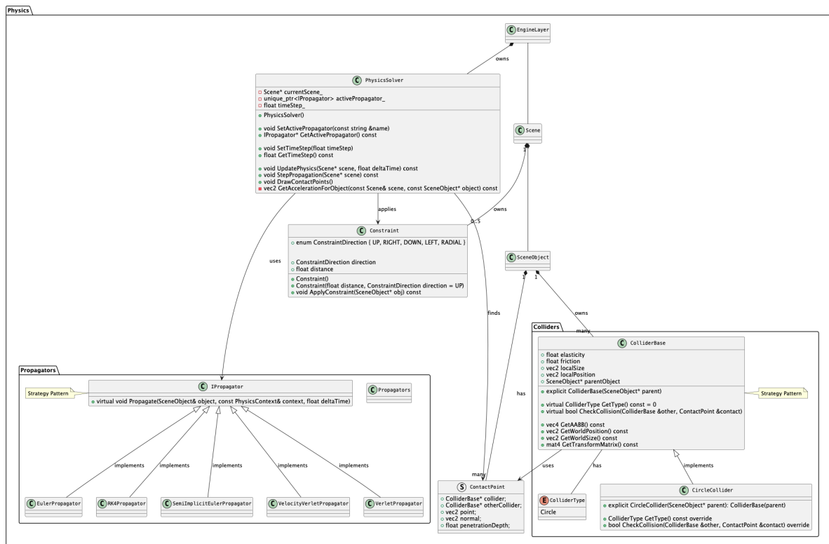
Abbildung 3: Überblick über die Struktur der Physik-Simulation, welche von der EngineLayer verwaltet wird
