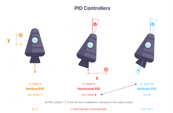
Abbildung 5: Regelungskonzept für die Schubvektorkontrolle
