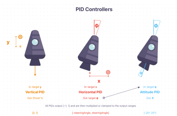
Abbildung 6: Regelungskonzept für die Schubvektorsteuerung
