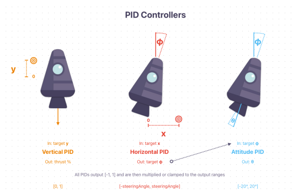
Abbildung 6: Regelungskonzept für die Schubvektorkontrolle
