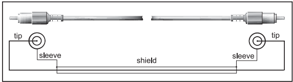
Fig. 4.1: RCA cable
