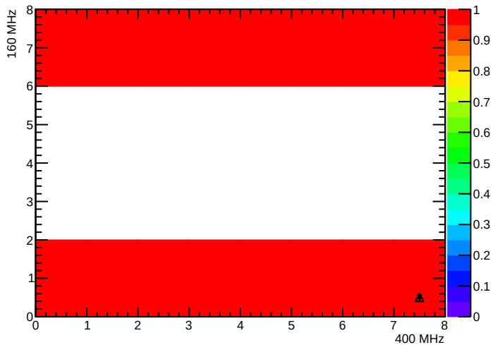
Bpix_BpI_SEC2_LYR3_LDR5F_MOD2_nROCHheaders
