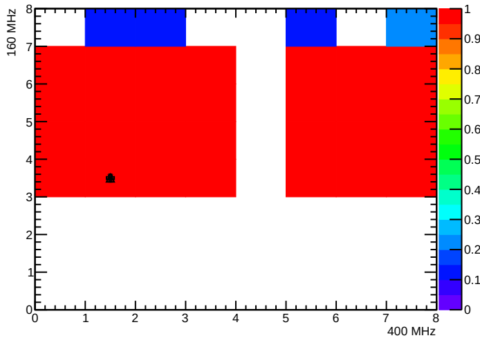
BPix_Bml_SEC2_LYR3_LDR3F_MOD2_nTBMDecodes
