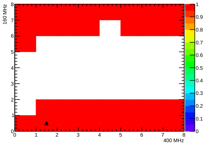
BPix_Bpl_SEC8_LYR3_LDR22F_MOD4_nROCHheaders
