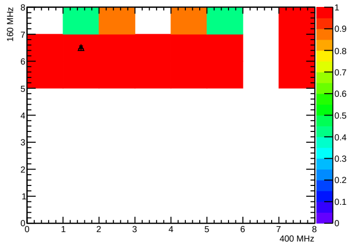
BPix_BpO_SEC2_LYR2_LDR3F_MOD3_nROCHheaders
