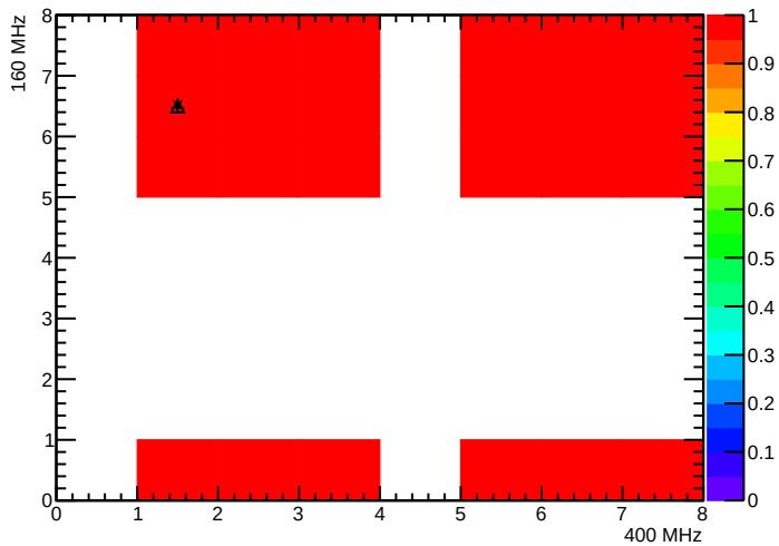
BPix_BpO_SEC3_LYR1_LDR2F_MOD1_nROCHheaders
