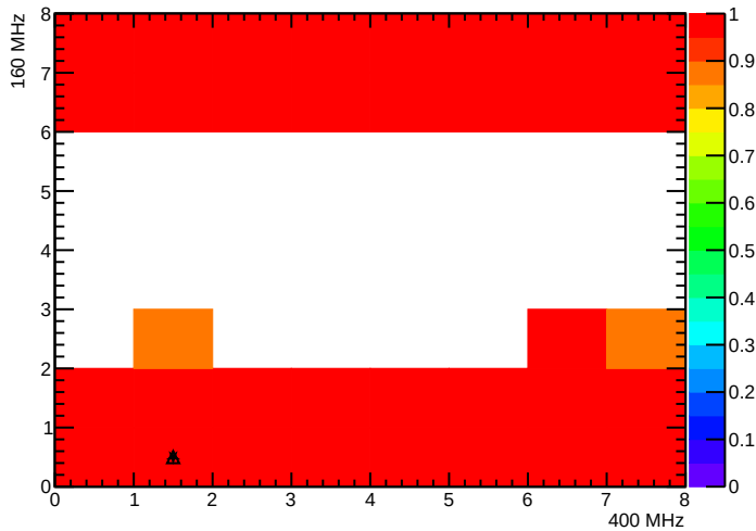
BPix_Bpl_SEC7_LYR4_LDR25F_MOD3_nROCHheaders
