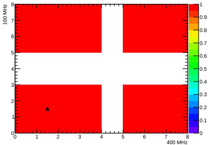
BPix_BpI_SEC1_LYR2_LDR2F_MOD2_nROCHheaders
