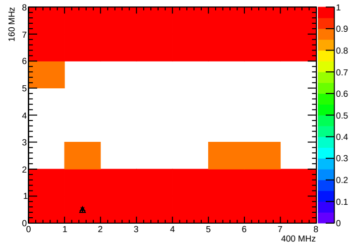
BPix_BpO_SEC7_LYR4_LDR25F_MOD4_nROCHheaders
