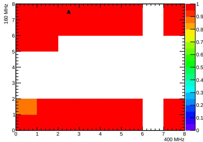
BPix_BpO_SEC4_LYR3_LDR9F_MOD1_nROCHheaders
