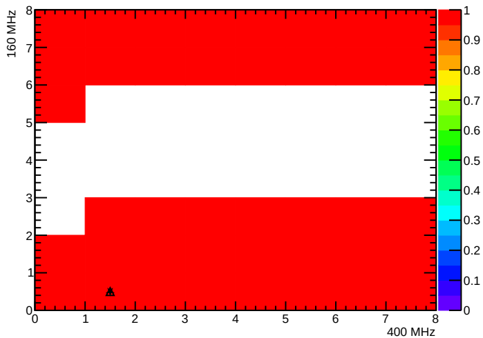
BPix_BpI_SEC3_LYR3_LDR8F_MOD1_nROCHheaders
