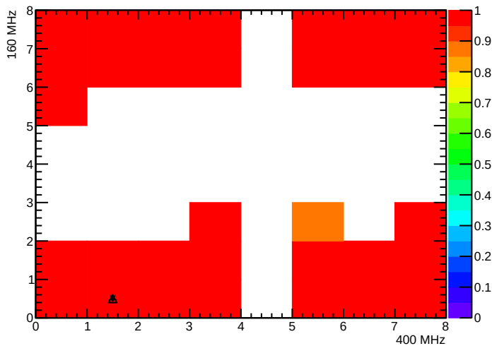
BPix_Bpl_SEC7_LYR4_LDR27F_MOD1_nROCHheaders
