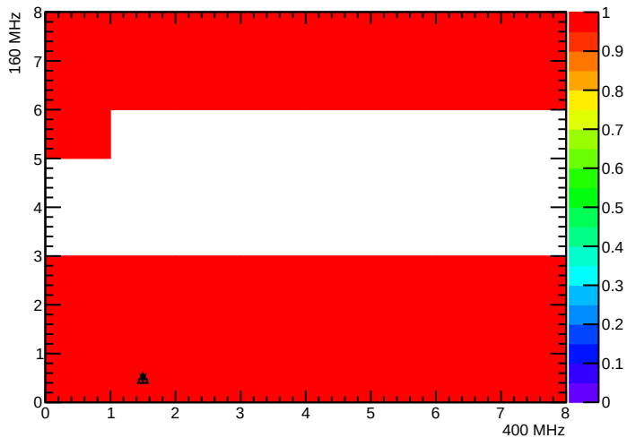
BPix_BpO_SEC8_LYR4_LDR32F_MOD3_nROCHheaders
