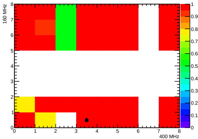
BPix_BpO_SEC2_LYR2_LDR4F_MOD3_nTBMDecodes
