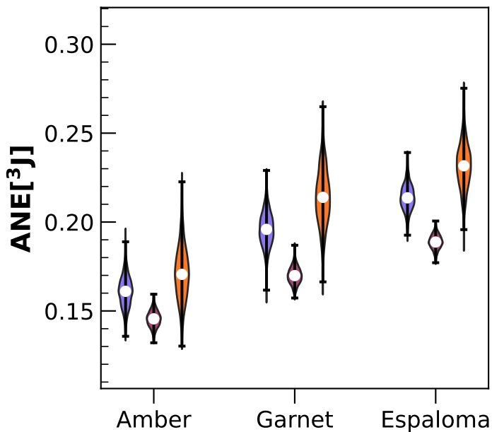
BPTI
