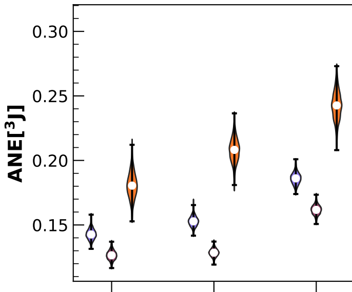
BPTI
