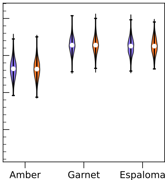
HEWL
