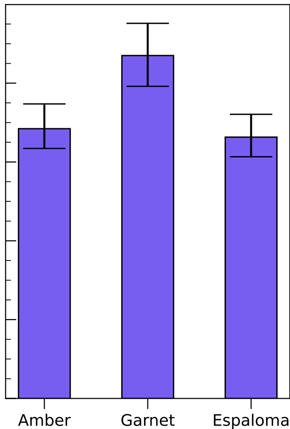
UBQ HBonds
