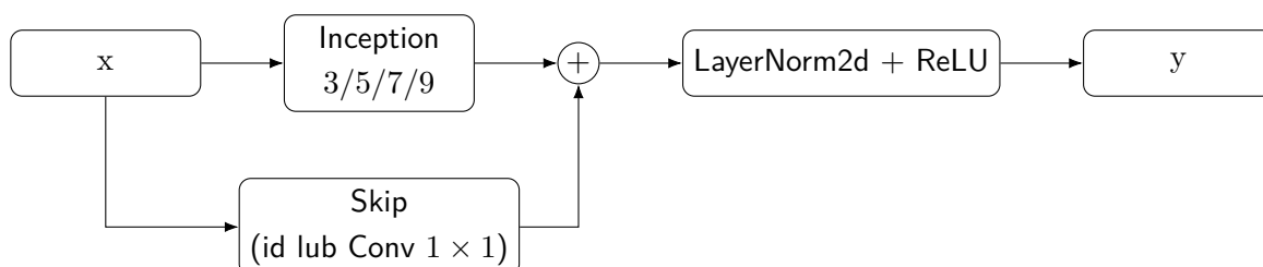
Rysunek 5. Schemat bloku Inception–Residual stosowanego w wariantcie residualnym.
