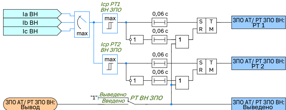
РТ ЗПО ВН 3561
