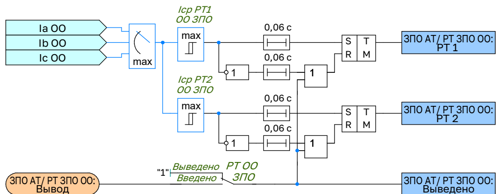
РТ ЗПО ОО 3562
