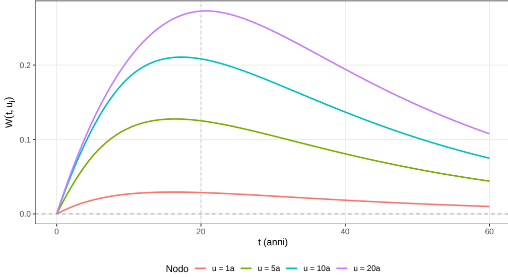
Figura 6: Funzioni di Wilson W(t, u_j) per u_j \in \{1, 5, 10, 20\} (4 dei m = 20 nodi di pagamento, scelti a scopo illustrativo). Ciascuna vale 0 in t = 0 e si smorza a zero per t \rightarrow \infty .
