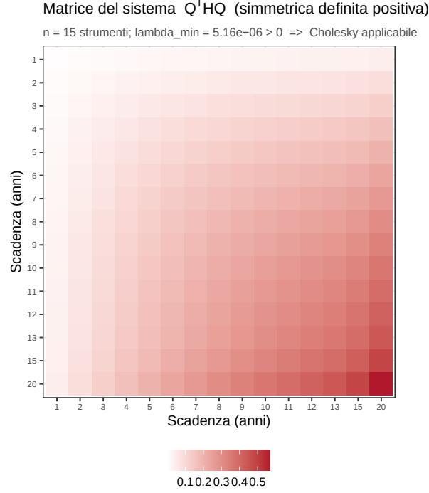
Figura 7: Matrice del sistema \mathbf{Q}^T \mathbf{H} \mathbf{Q} ( n = 15 ), dicembre 2025. È simmetrica e definita positiva ( \lambda_{\min} > 0 ): la fattorizzazione di Cholesky è applicabile ed è circa due volte più efficiente di una LU generica.
