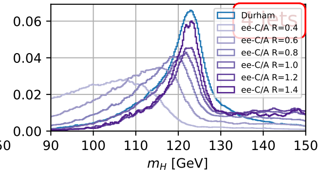
Z(\rightarrow bb)H(\rightarrow gg)
