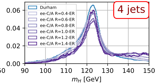
Z(\rightarrow bb)H(\rightarrow bb)
