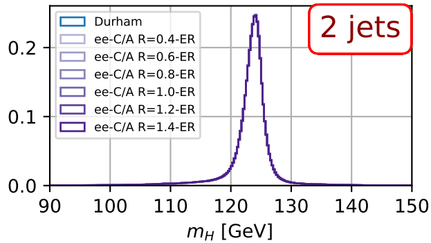
Z(\rightarrow\nu\nu)H(\rightarrow gg)
