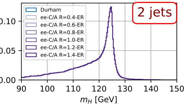
Z(\rightarrow\nu\nu)H(\rightarrow bb)
