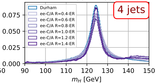
Z(\rightarrow qq)H(\rightarrow gg)
