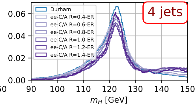
Z(\rightarrow qq)H(\rightarrow bb)
