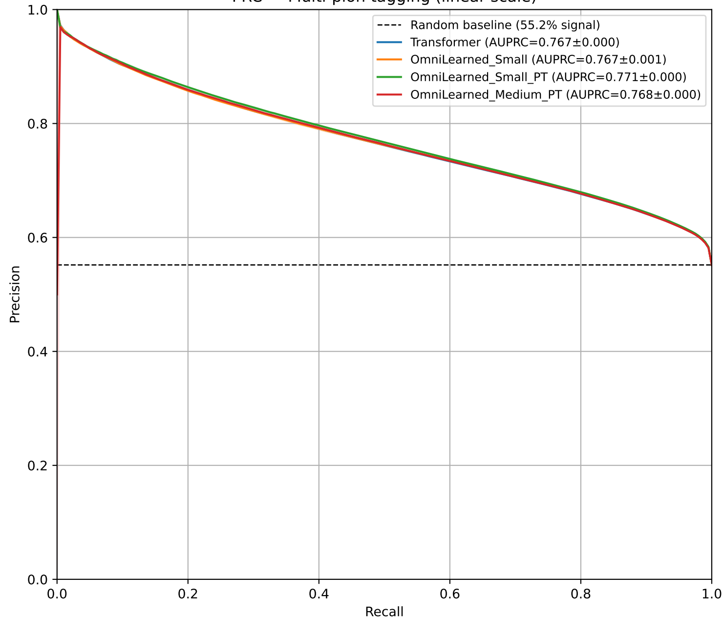
PRC — Multi-pion tagging (linear scale)
