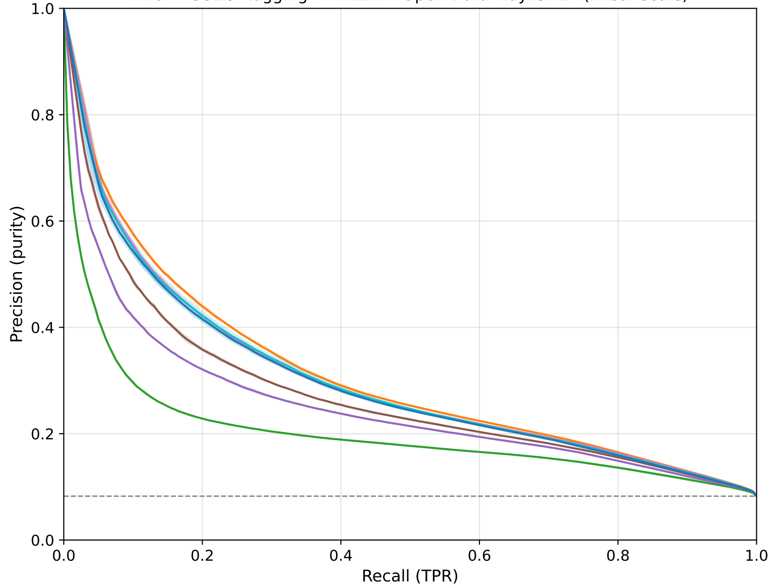
PRC — CC1\pi^0 tagging - MINERvA Open Data Playlist 1A (linear scale)
