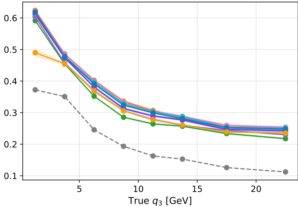
AUPRC vs. True q_3
