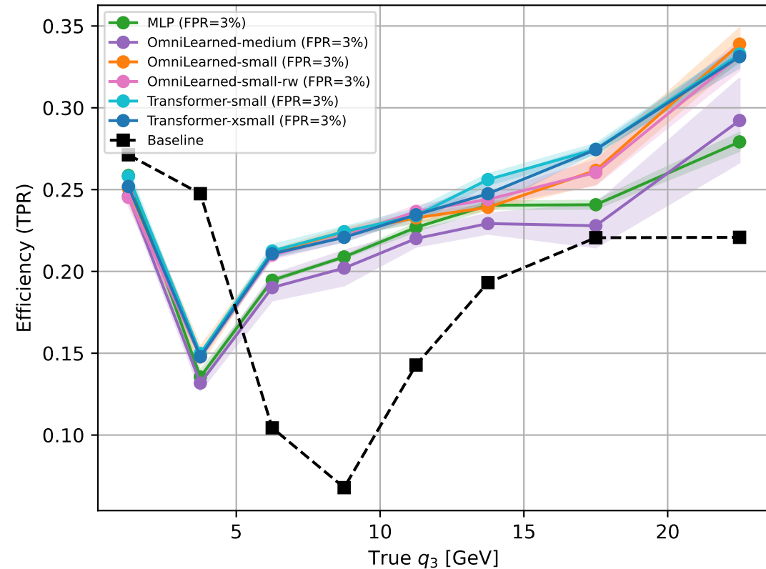
TPR @ fixed FPR vs. True q_3
