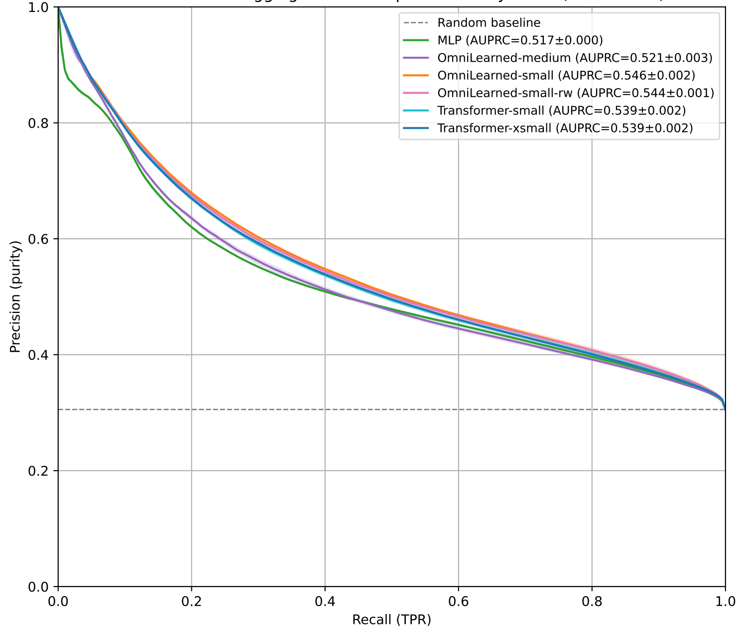
PRC — CC1\pi^\pm tagging - Minerva Open Data Playlist 1A (linear scale)
