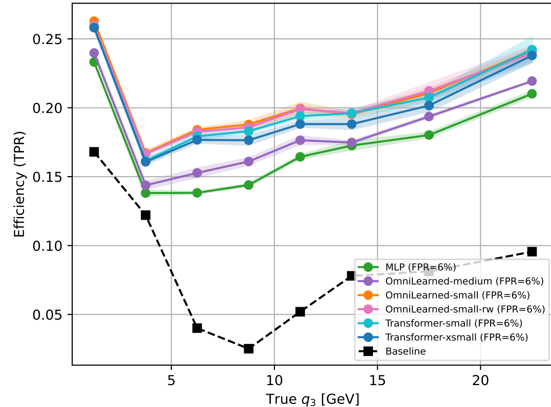
TPR @ fixed FPR vs. True q_3
