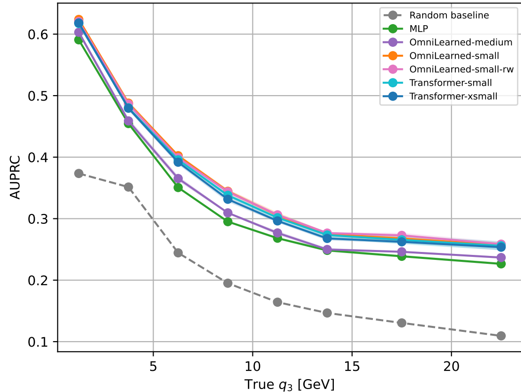
AUPRC vs. True q_3
