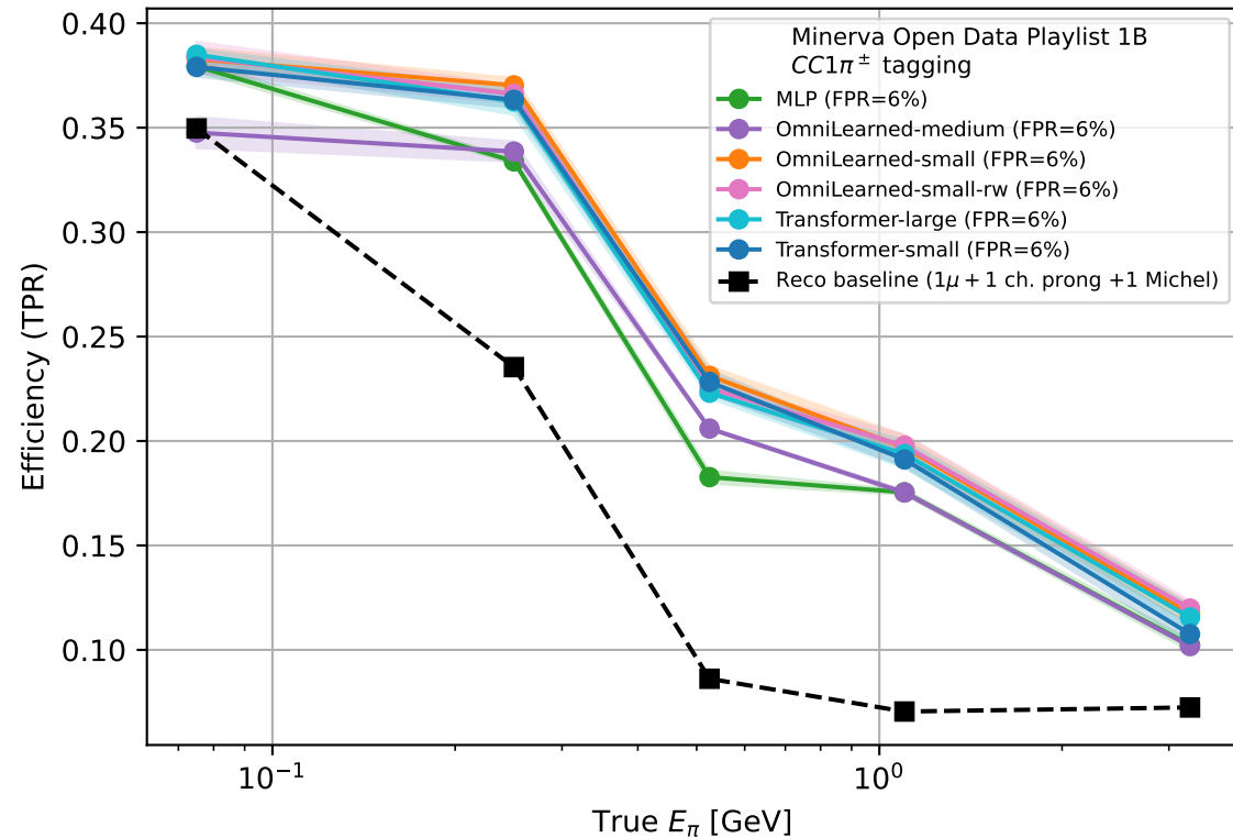
TPR @ fixed FPR
