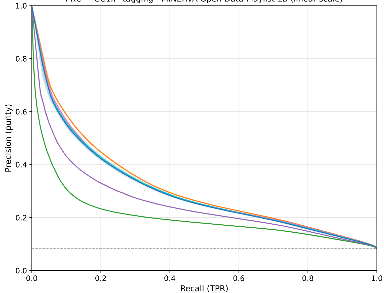
PRC — CC1\pi^0 tagging - MINERvA Open Data Playlist 1B (linear scale)
