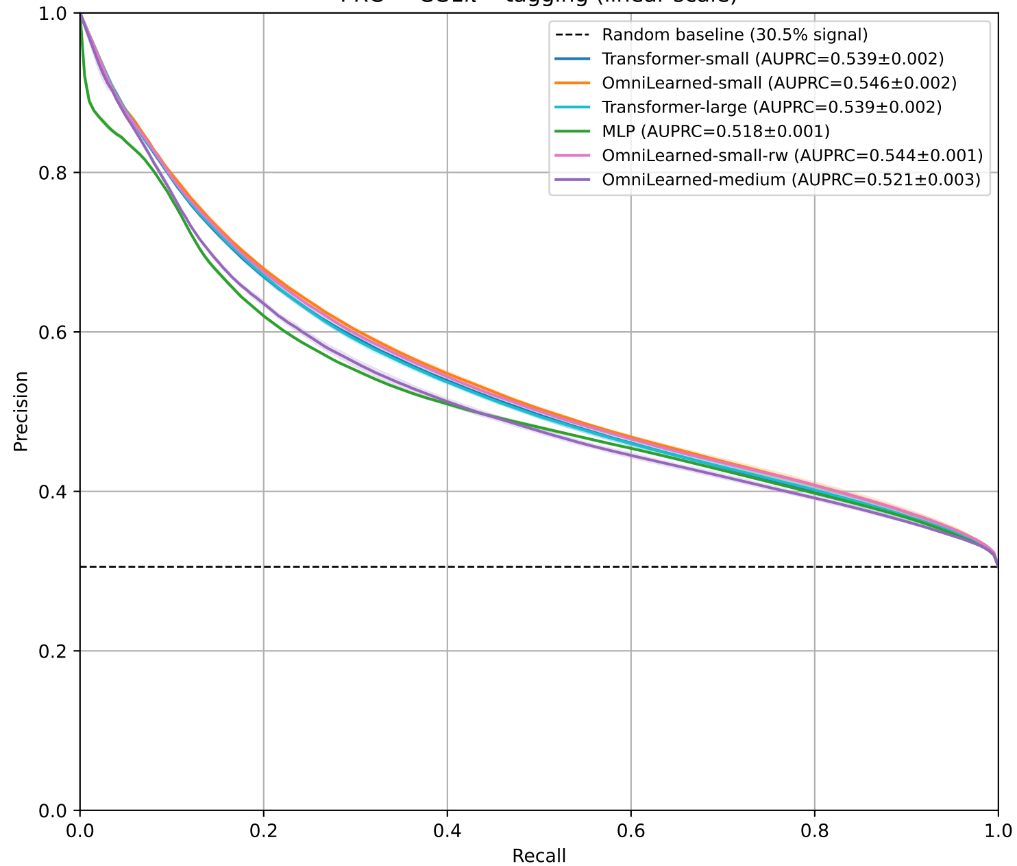
PRC — CC1\pi^\pm tagging (linear scale)
