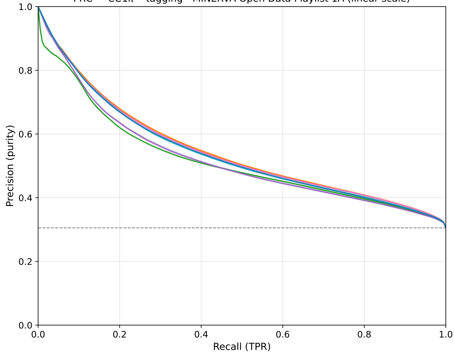
PRC — CC1\pi^\pm tagging - MINERvA Open Data Playlist 1A (linear scale)
