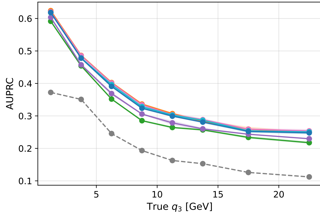
AUPRC vs. True q_3
