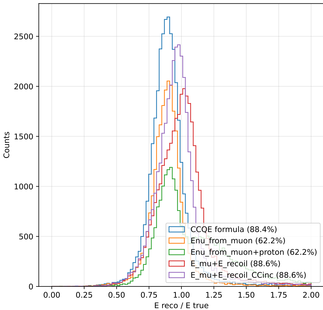
E reco / E true Distribution - RES
