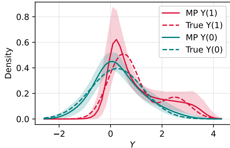
S-Learner
