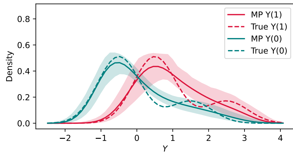
Scenario 2: S-Learner
