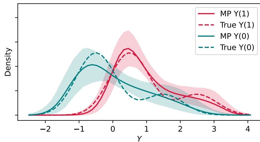
Scenario 2: T-Learner
