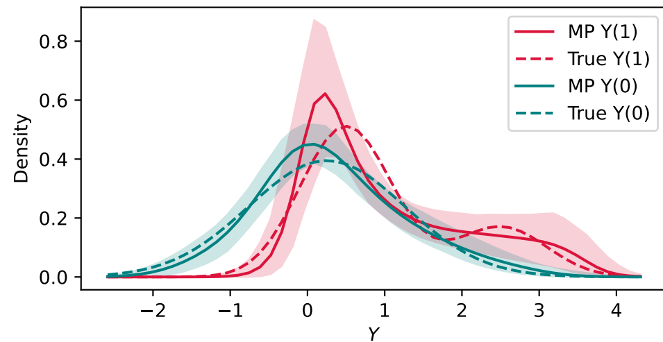
Scenario 1: S-Learner
