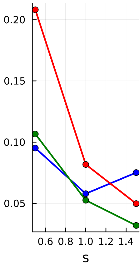
MAE
