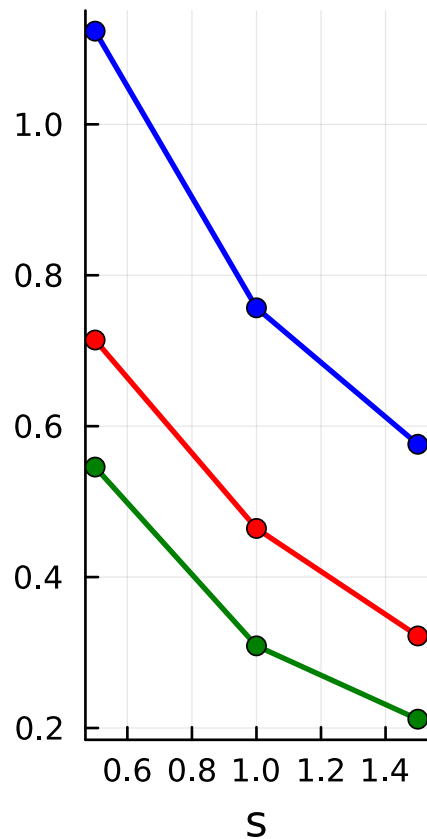
MIL
