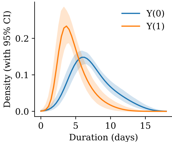
S-Learner
