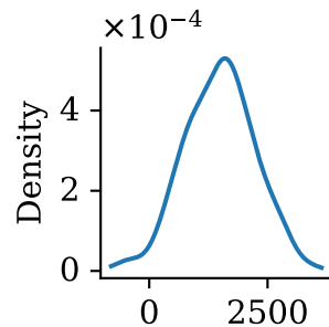
ATT
