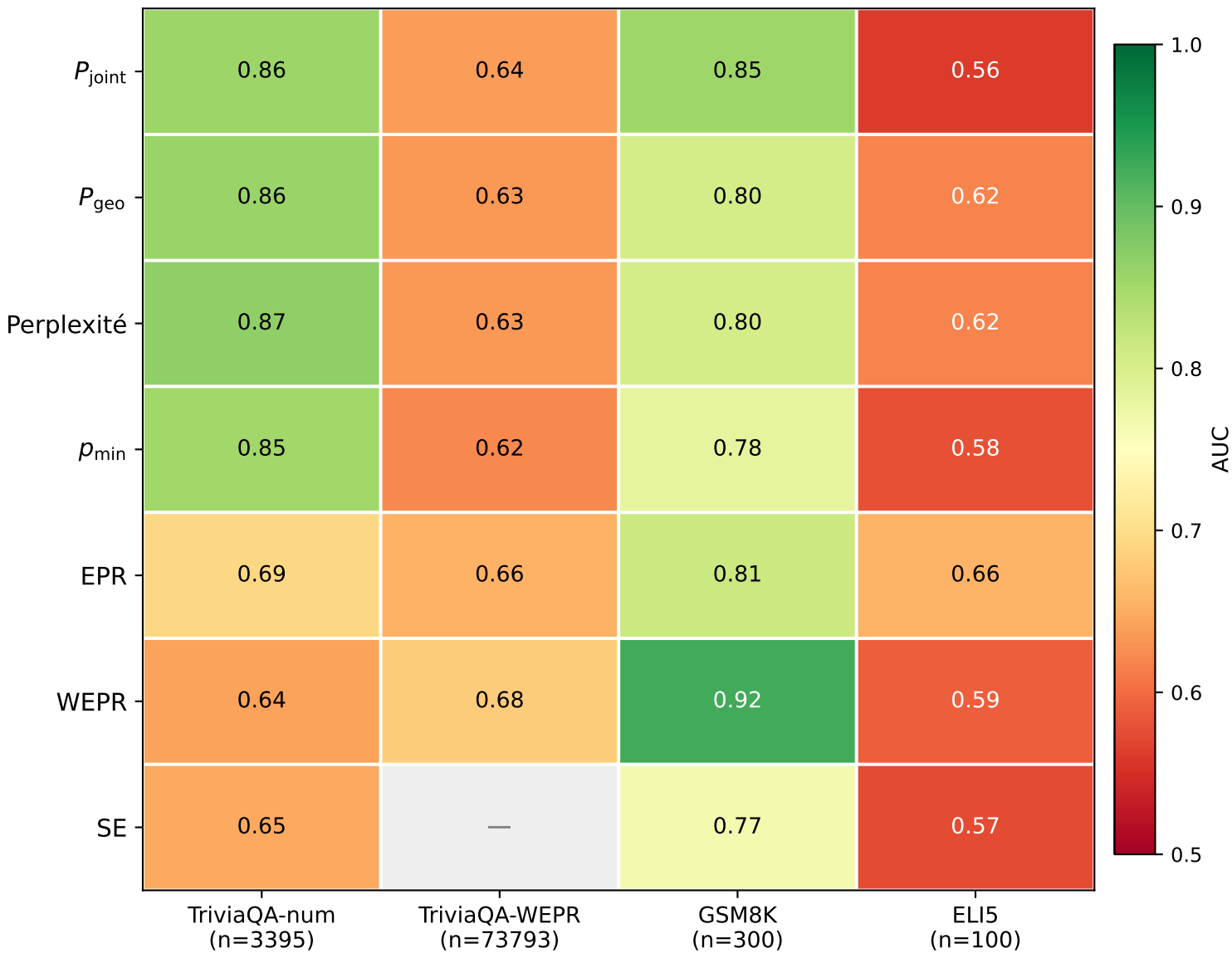
AUC de discrimination correct/incorrect par dataset
