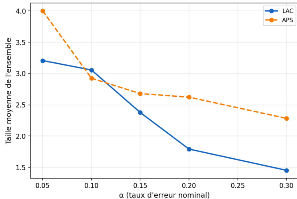
Taille d'ensemble vs \alpha
