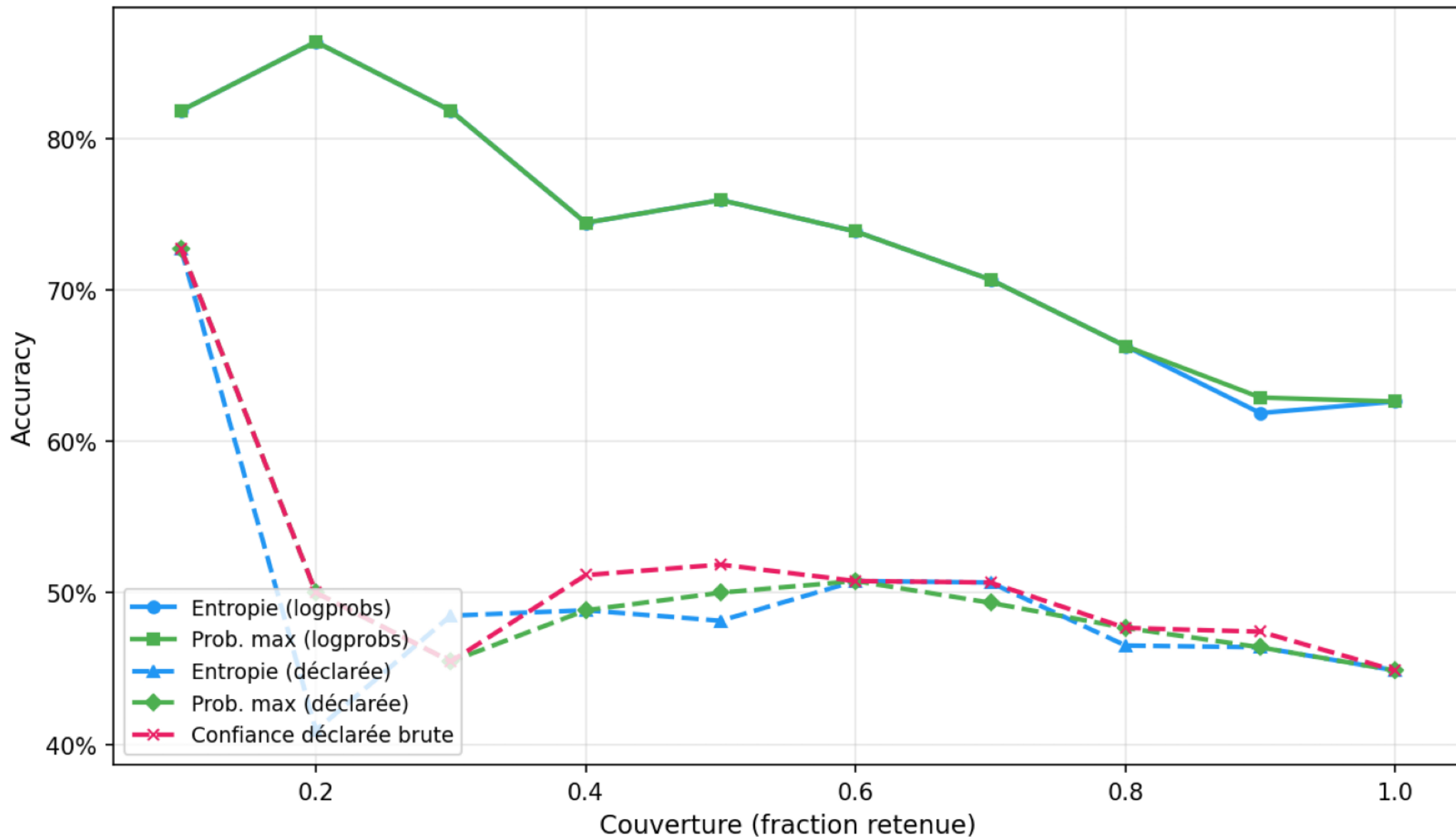
Accuracy vs Couverture — Logprobs vs Déclarée (n=107)
