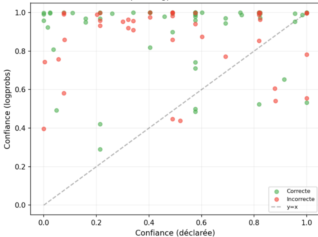
Entropie : Logprobs vs Déclarée
