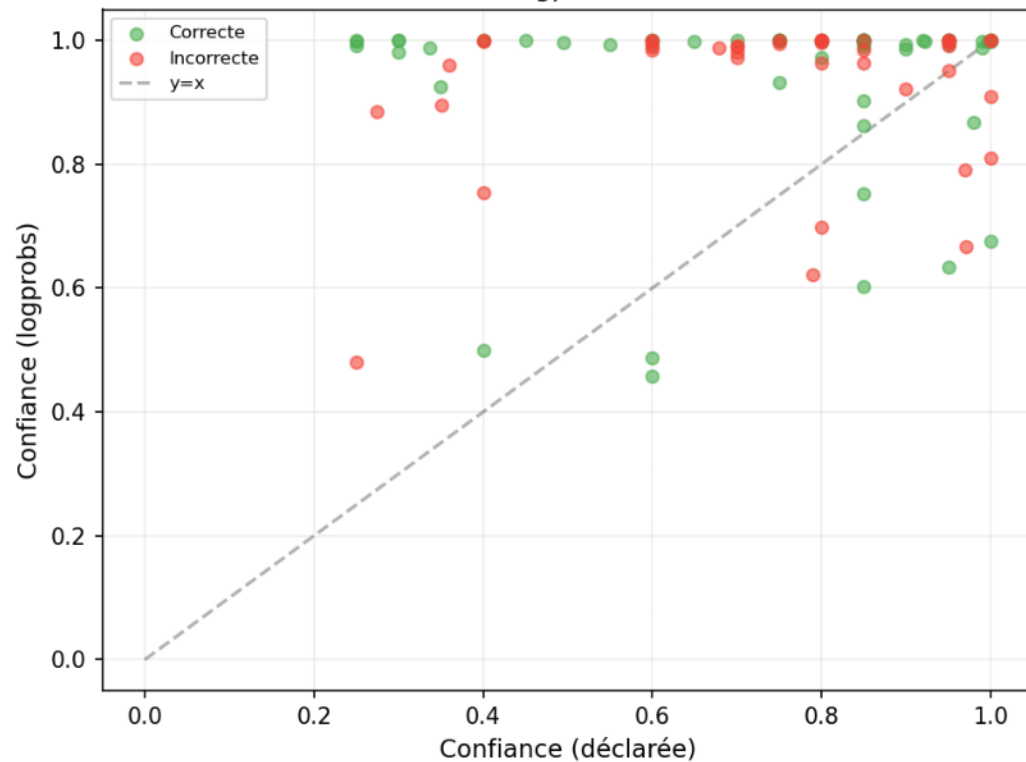
Prob. max : Logprobs vs Déclarée
