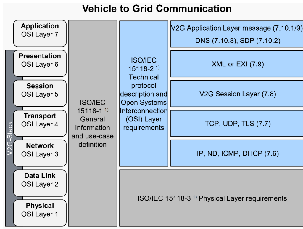
Abbildung 2.4: V2G OSI [3, S. 43]
