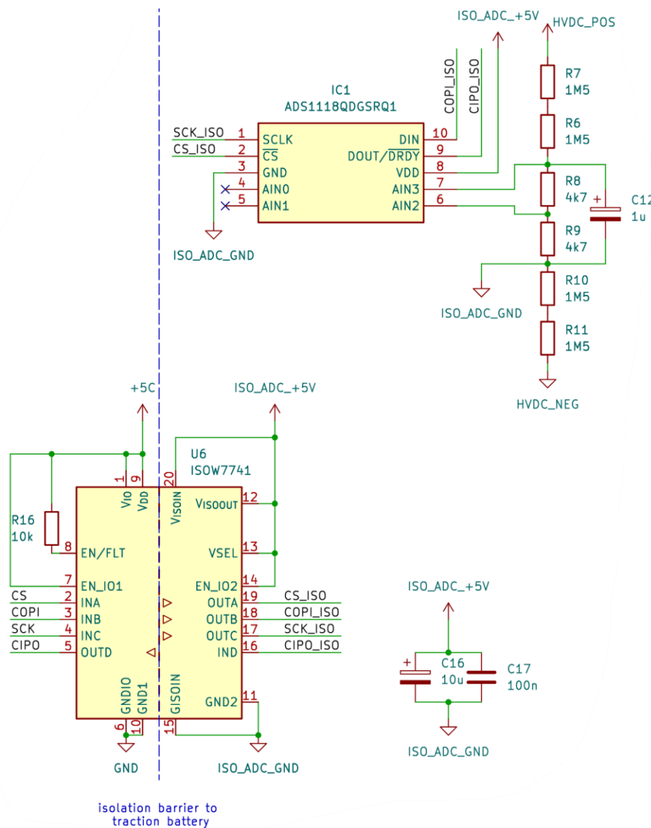
Abbildung 3.5: Schaltplan zur Spannungsmessung
