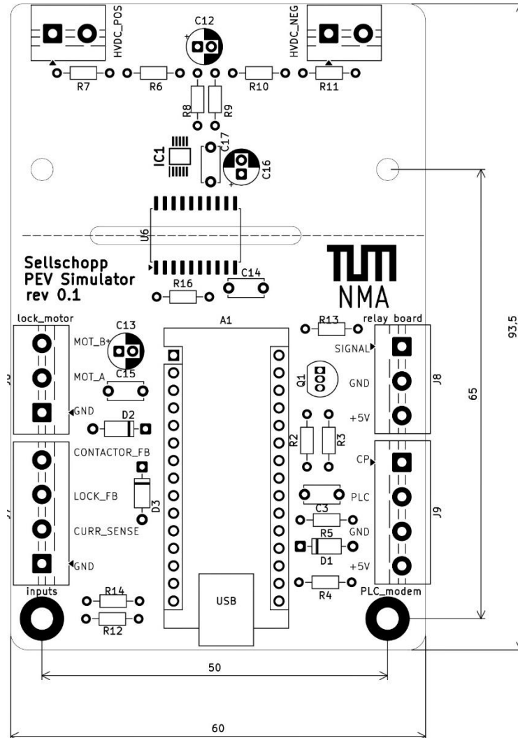
Abbildung C.1 Maße Platine
