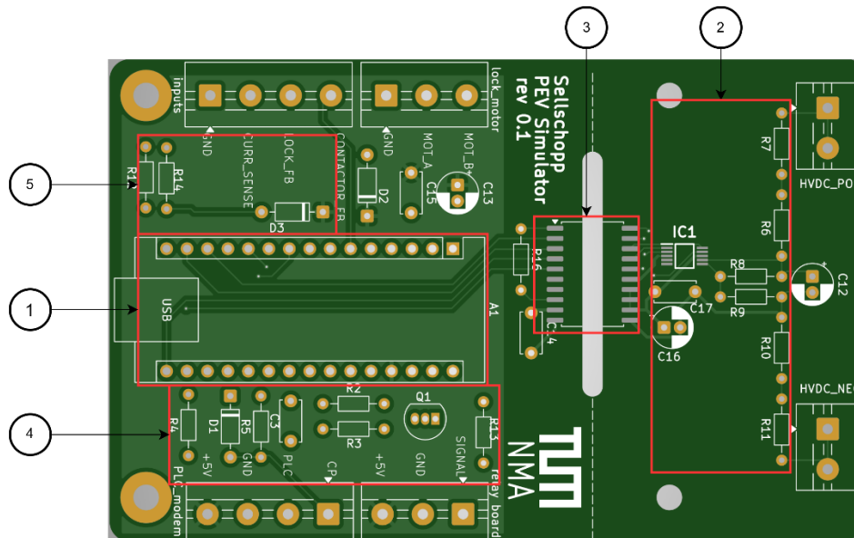
Abbildung 3.6: Visualisierung des PCB
